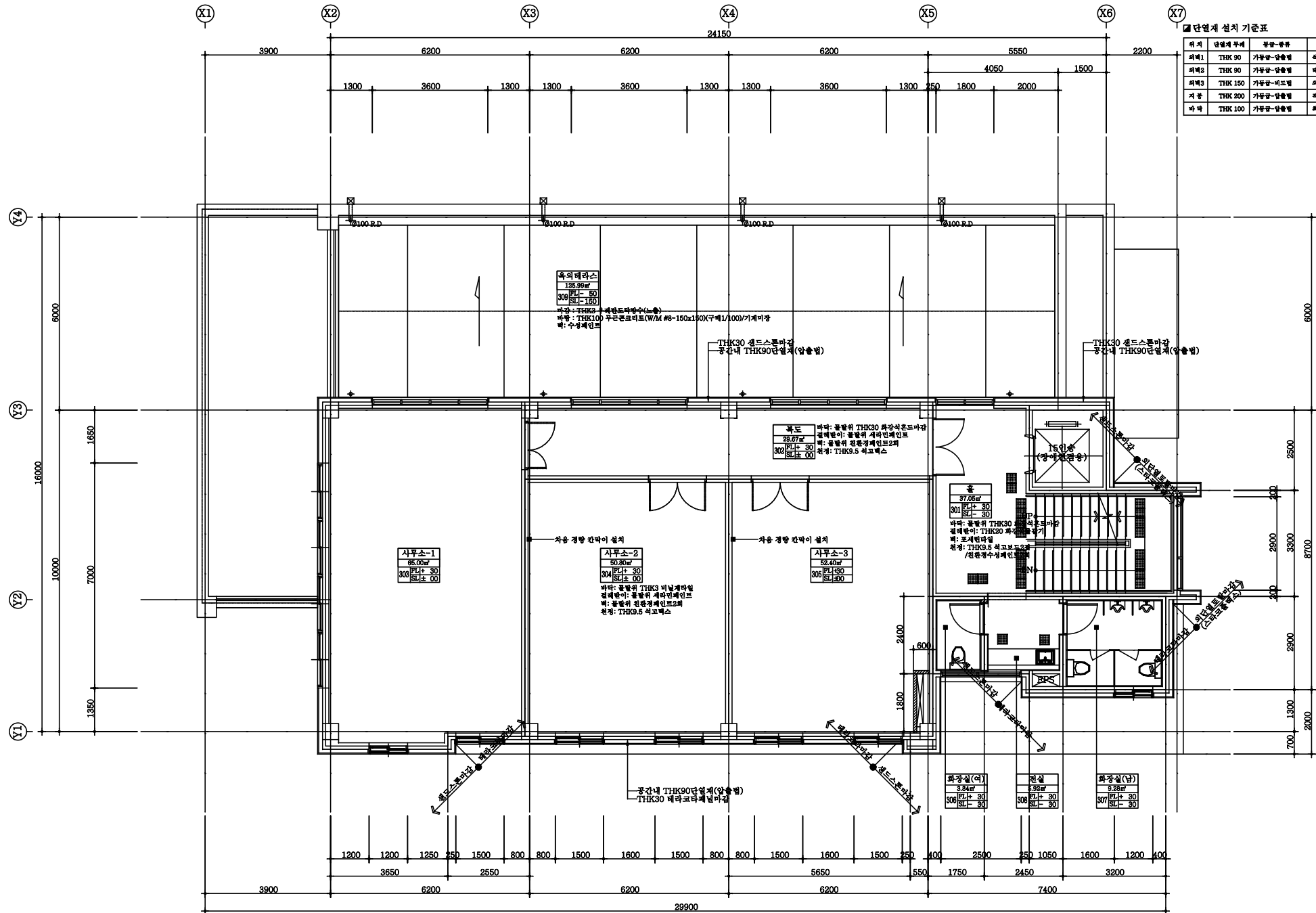
1 3층 평면도 SCALE(A3) : 1/120
