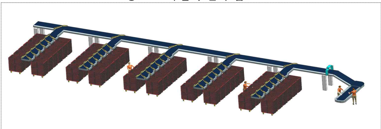
<소형 소포 구분기 설치 참조도>
